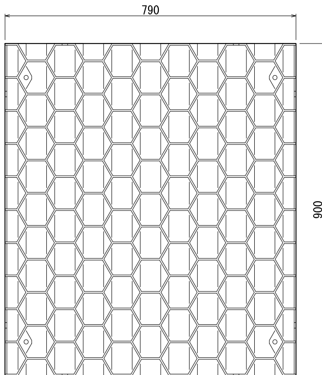
平面図
