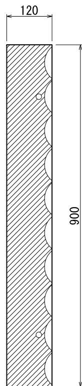
側面図
